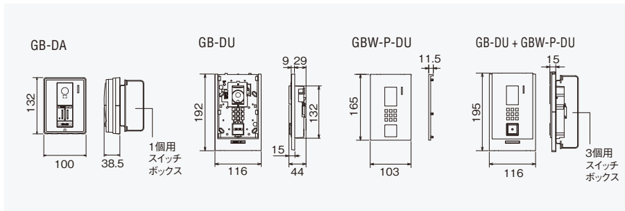
カメラ付玄関子機 GB-DA 希望小売価格 46,000 円(税別) ●住戸アダプター内蔵
