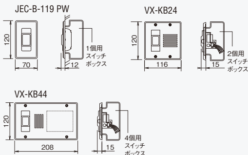
■寸法図(mm)
