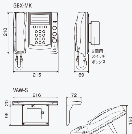
■寸法図(mm)
