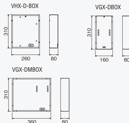
■寸法図(mm)
